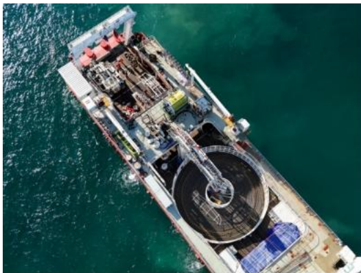
SEA-H2X 项目中国海南登陆现场
