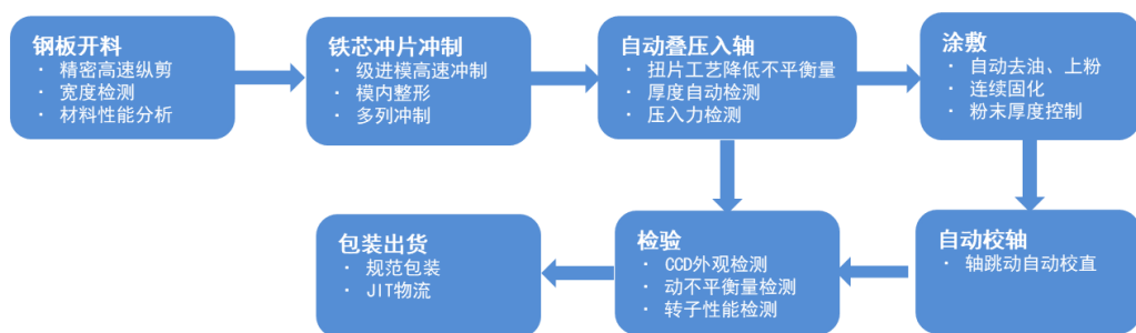
(2) 微特电机转定子铁芯工艺流程图
