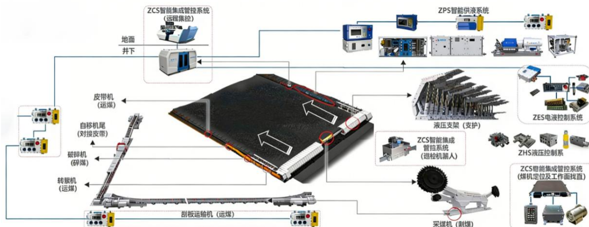
图 5 四大系统与煤矿综采工作面设备对应关系示意图
