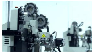
智能绕线机器人
